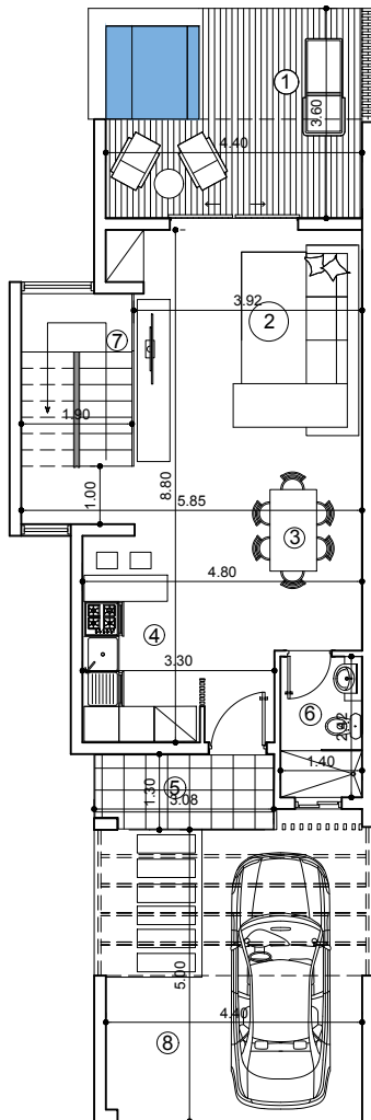
PLANTA DIMENSIONADA 1ER PISO
