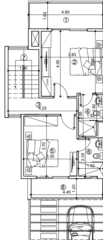
PLANTA DIMENSIONADA 2DO. PISO
