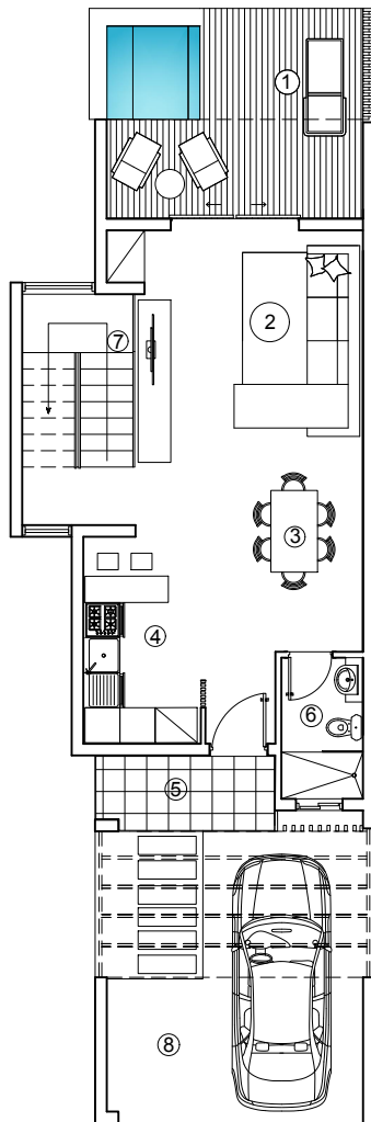
PLANTA ARQUITECTONICA 1ER PISO
